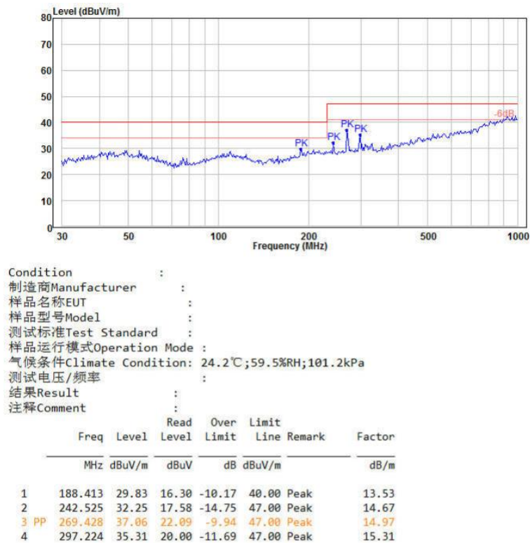
图 6-5 RE 测试水平方向
