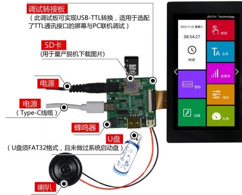
图 1-4 调试工具图
