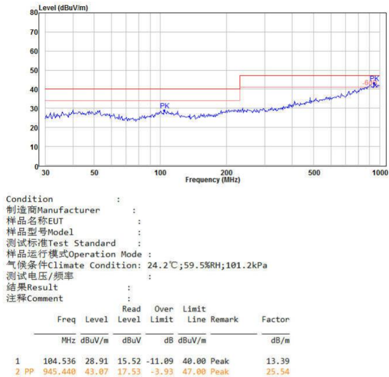
图 6-6 RE 测试垂直方向
