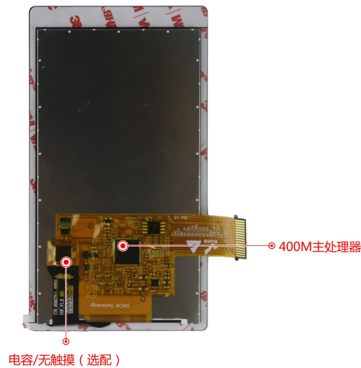
图 1-3 硬件配置图
